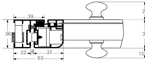
Detalle de cierre
